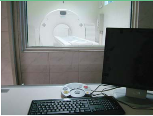
O tomógrafo da Santa Casa, no dia em que chegou e montado em sala apropriada no CEDISC, no mês de fevereiro
